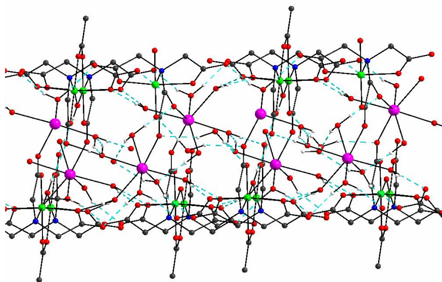
Fig. 2. Stratul 2D în structura compusului [\text{CaCr}_2(\mu\text{-OH})(\mu\text{-OAc})(\text{nta})_2 \cdot 6\text{H}_2\text{O}] \cdot 2\text{H}_2\text{O} (atomii de hidrogen ce nu fac parte din legăturile de hidrogen sunt omise pentru claritate)
